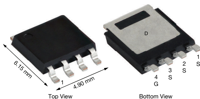
PowerPAK® SO-8L
