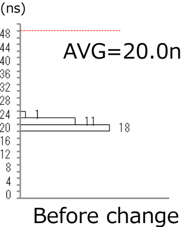
|tpHL-tpLH| (IF=0↔10mA, VCC2=20V, Rg=10Ω, Cg=25nF)
