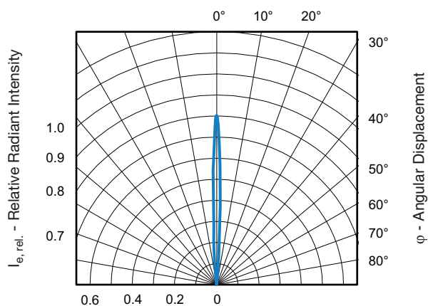
Fig. 6 - VCSEL Profile
