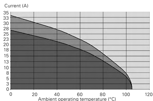
Fig.3: UTGX 12-4 – Wire section 20 AWG
