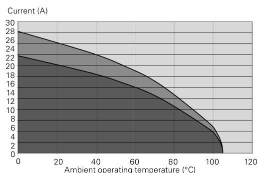
Fig.1: UTGX 12-4 – Wire section 16 AWG
