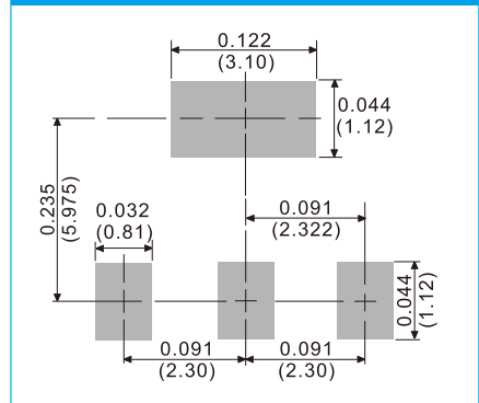
SOT-89
