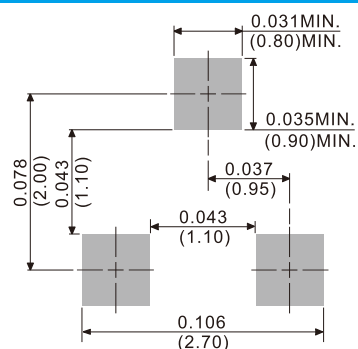
SOT-23
