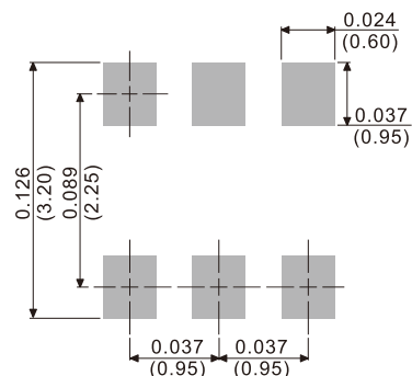
SOT-23 6L
