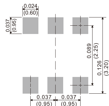
SOT-23 6L-1/SOT-26-1
