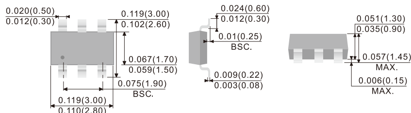
SOT-23 6L-1/SOT-26-1
