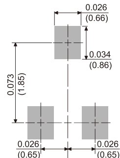
SOT-323
