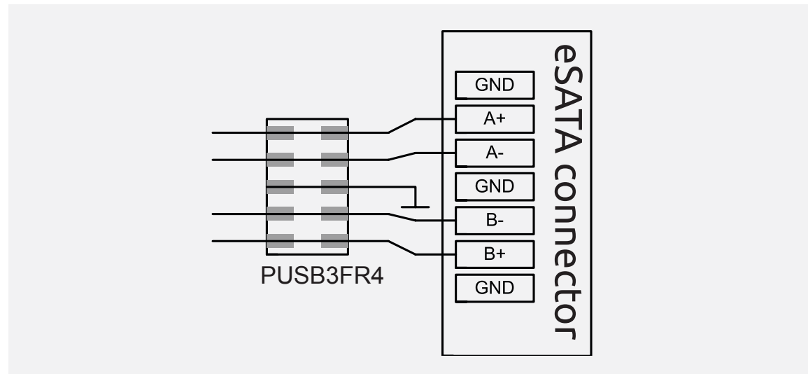
eSATA ESD protection using PUSB3FR4
