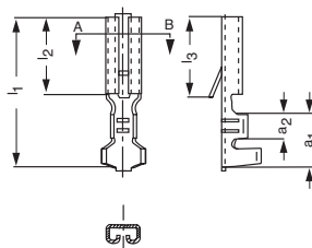
Schnitt A-B
