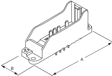
Flachsteckerwanne 2,8 x 0,8 mm
