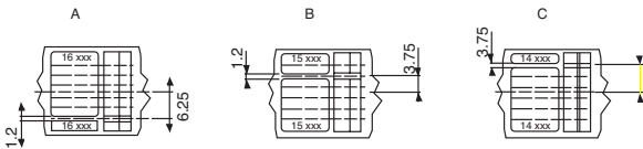
Flachsteckerwanne 2,8 x 0,8 mm
