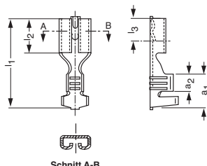
Schnitt A-B
