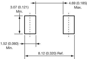
DO-214AB (SMC)
