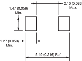
DO-214AC (SMA)
