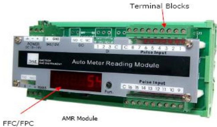
AMR Module
