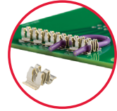
Griplet™ Miniature IDC
