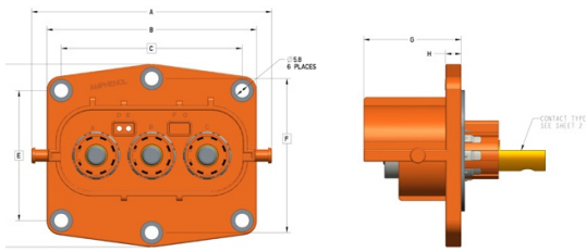
3-Pole Receptacle 3芯插座
