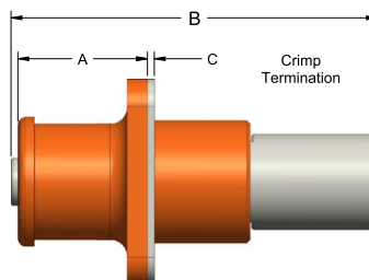
压接接线
