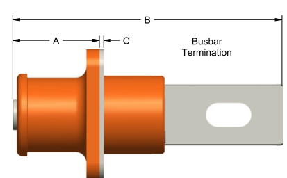
汇流排接线
