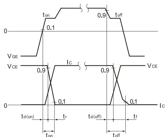
図 2. スイッチング時間波形 Fig 2. Switching Time Waveforms
