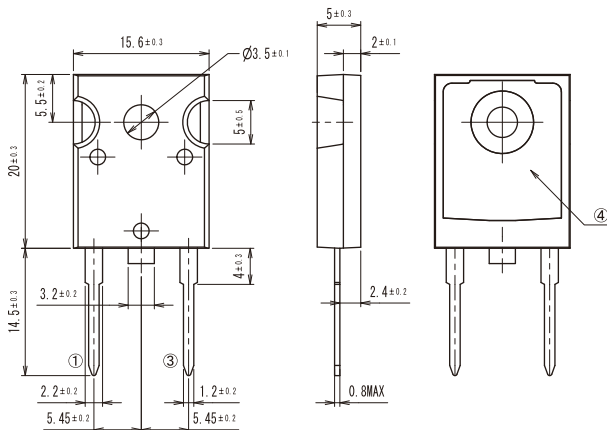
<A-23> TO-247 2pin
