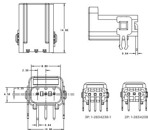
Receptacle
