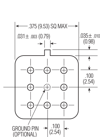
Header
