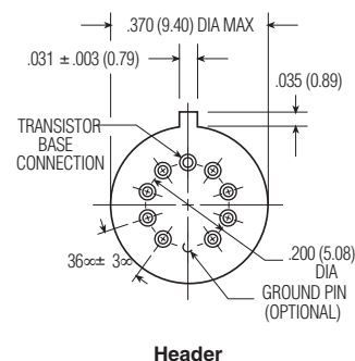
Header
