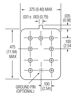
MGST Header
