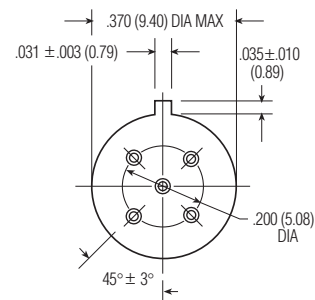
1MA/1MAD/1MADD Header
