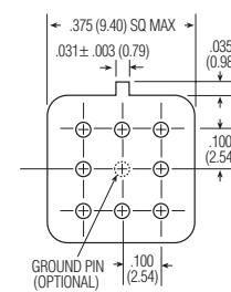
MGS/MGSD/MGSDD Header
