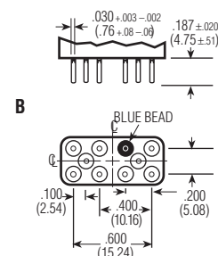
LS Terminals
