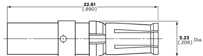
Socket
