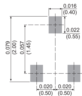
SOT-523
