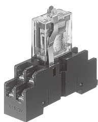
NC2 DIN terminal socket
