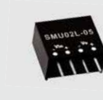
▲ SMU02 0.46" x 0.3" x 0.4"
