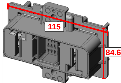
Receptacle
