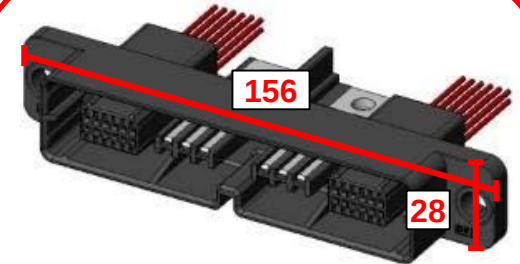
Receptacle
