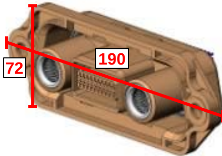
Receptacle
