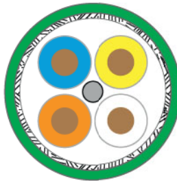
S/UTQ (Quad)
