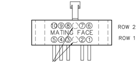
RECEPTACLE MA-281-010-435-ALC00
