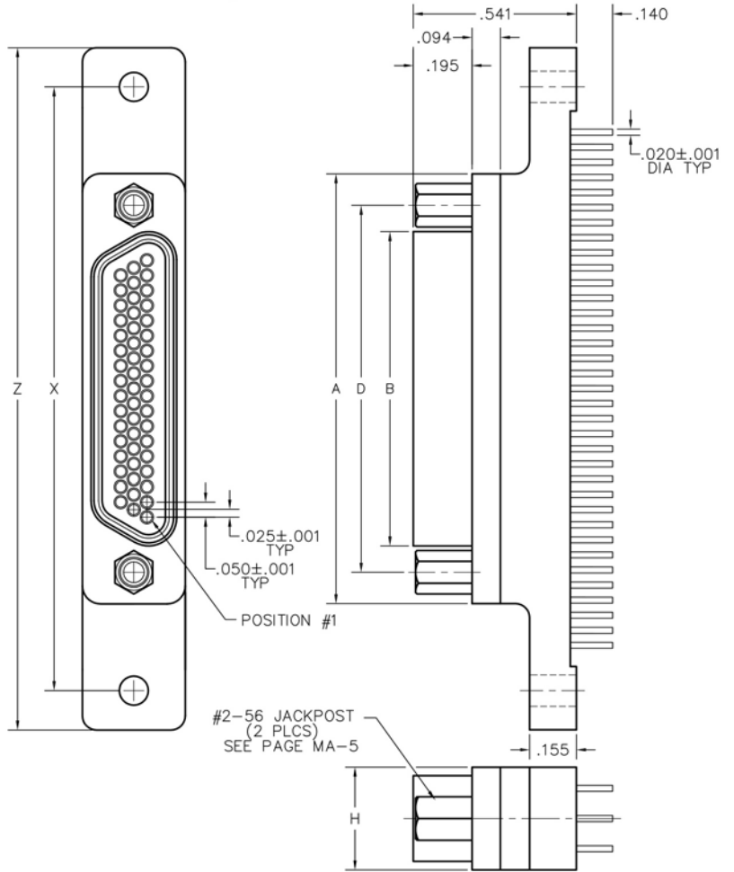
RECEPTACLE
