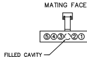
RECEPTACLE MA-141-005-261-A03WA
