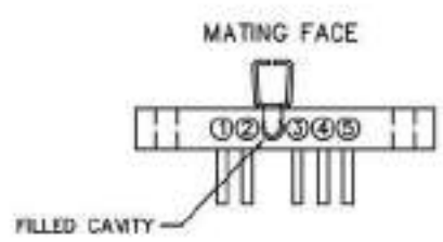
PLUG MA-171-005-325-A0300
