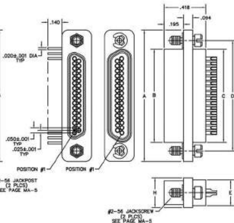
RECEPTACLE
