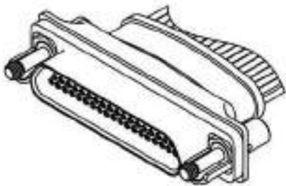
MM-2Q2-031-201-99WA-KS11 (RECEPTACLE)
