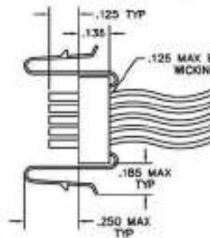
RECEPTACLE
