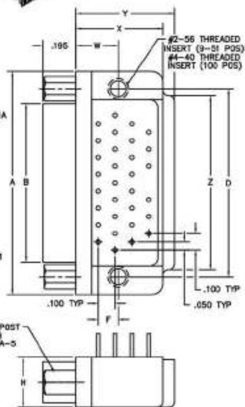
RECEPTACLE
