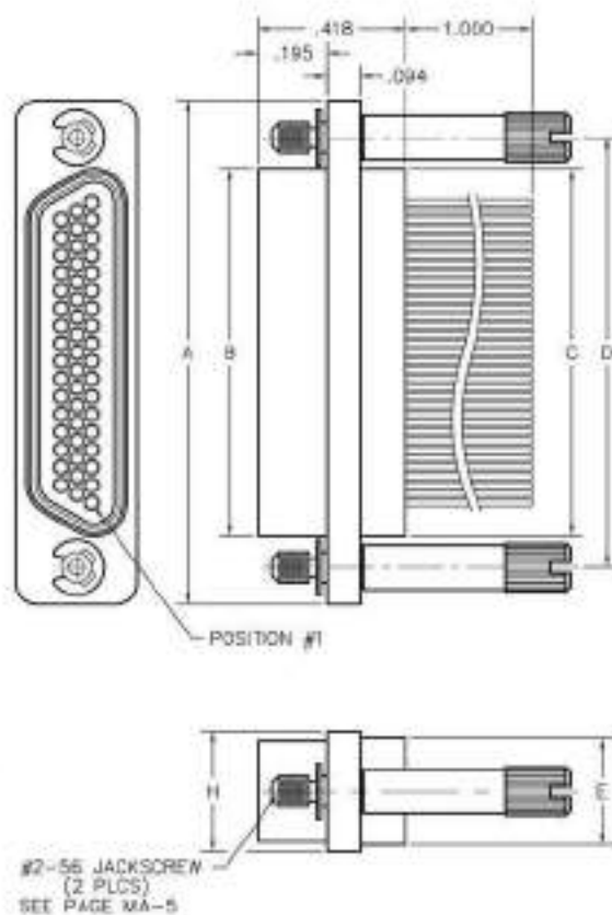
RECEPTACLE
