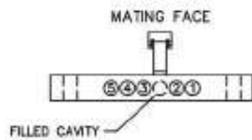
RECEPTACLE MA-121-005-261-A03WA
