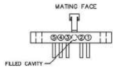
RECEPTACLE MA-181-005-435-A0300
