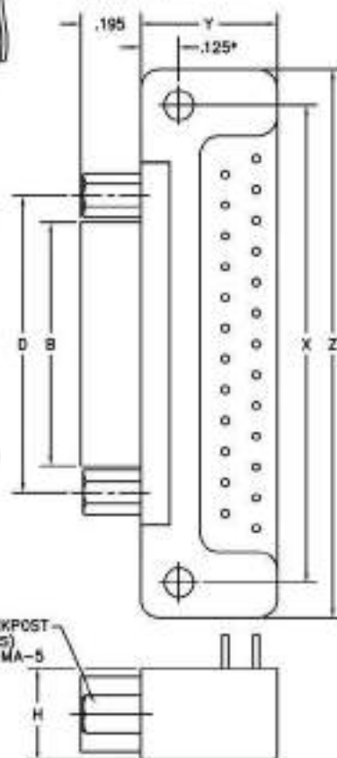
RECEPTACLE
