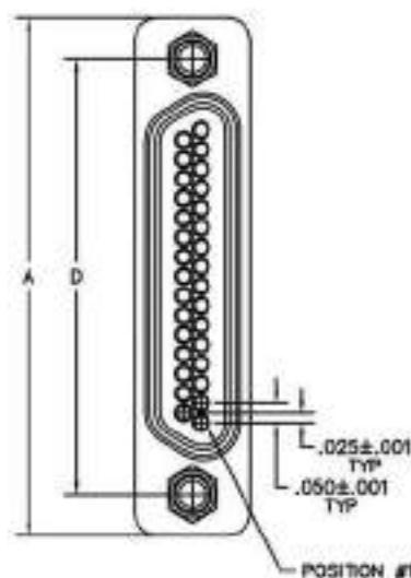
RECEPTACLE
